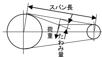
Vベルトの適当な張り強さ
